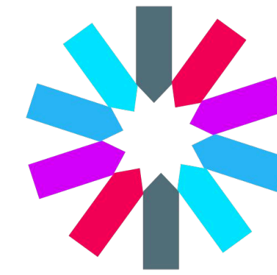
JWT & OAuth2
