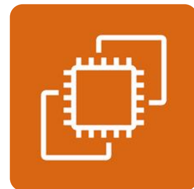
AWS EC2
