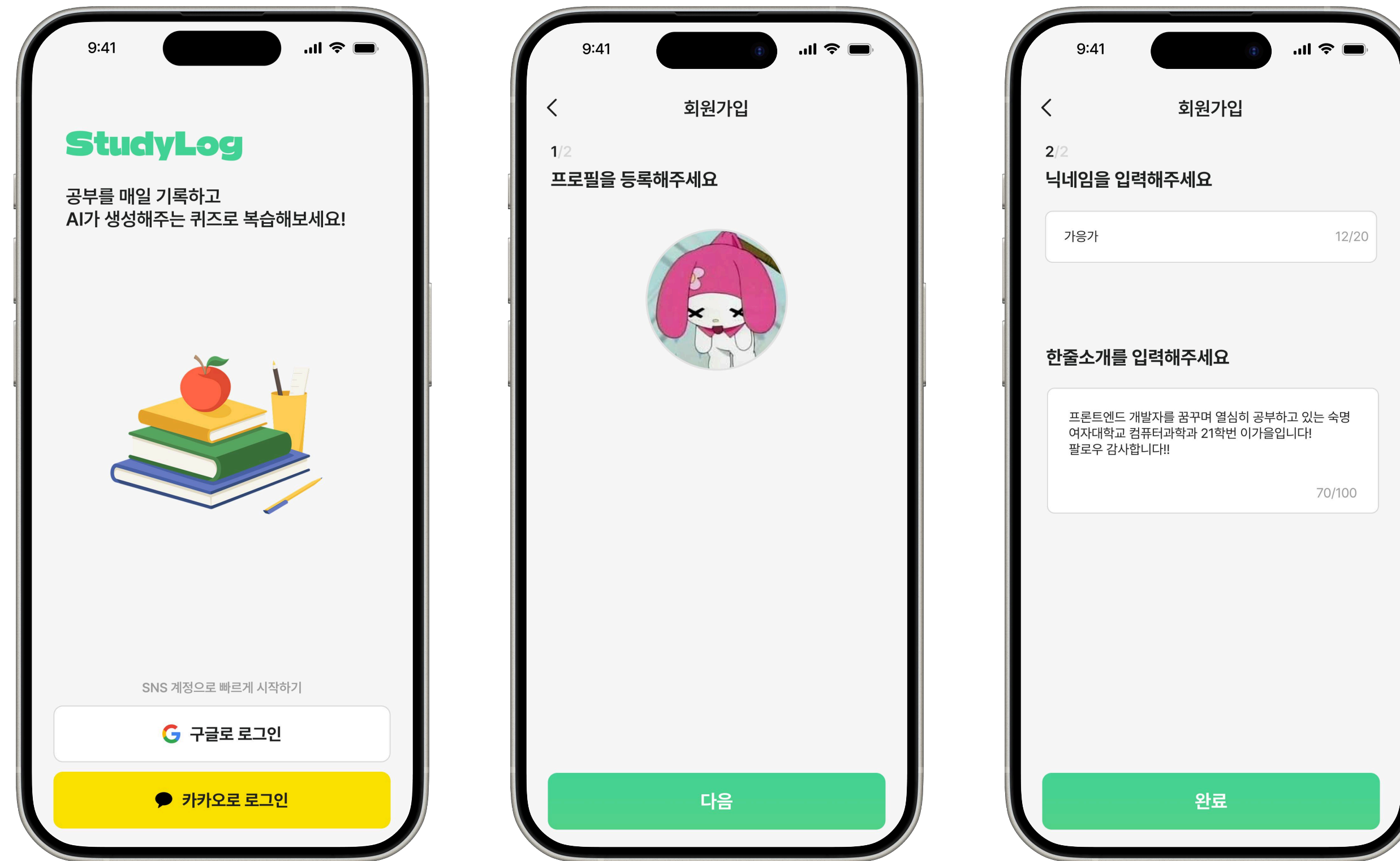
OAuth2.0 + JWT 기반 소셜 로그인 구현 Redirect URL로 사용자 인증 후 사용
