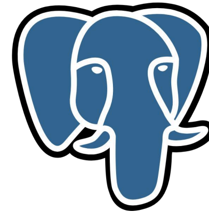
PostgreSQL
